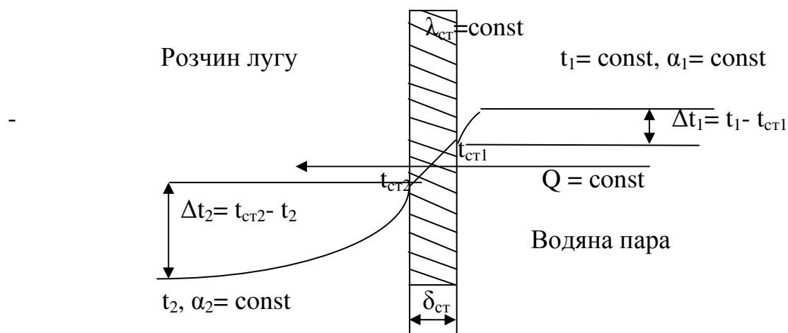
Рисунок 6.1. Розрахункова схема процесу теплопередачі.
