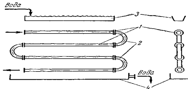
1 – секції прямих труб; 2 – калачі; 3 – розподілювальний жолоб; 4 – піддон Рисунок 1.6 – Схема зрошувального теплообмінника
