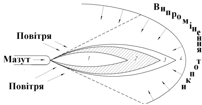
Рис. 3.4. Спалювання за допомогою форсунок
