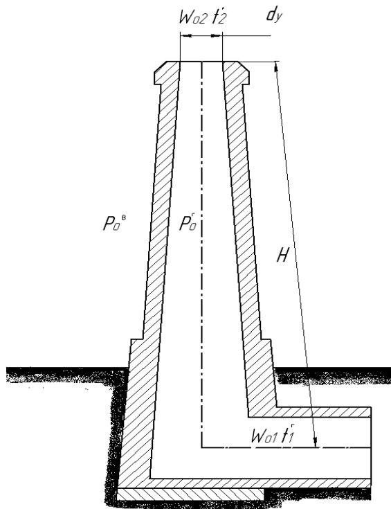
Рис. 5.1. Схема димаря
