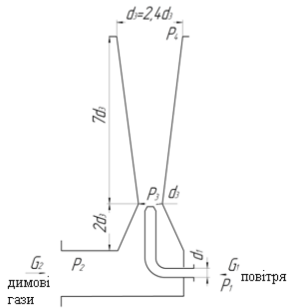
Рис. 5.3. Схема ежектора
