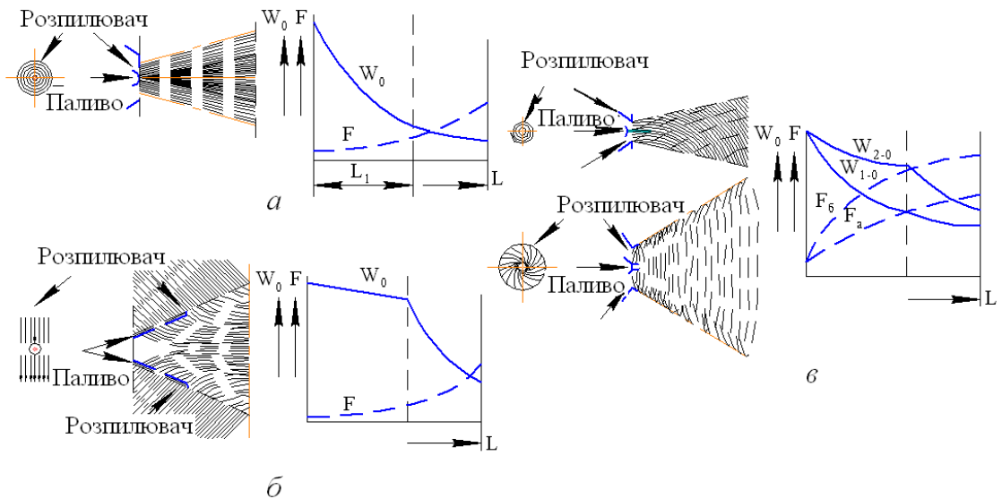
а - прямопотокове розпилення; б - розпилення зустрічними потоками; в - вихрове розпилення
