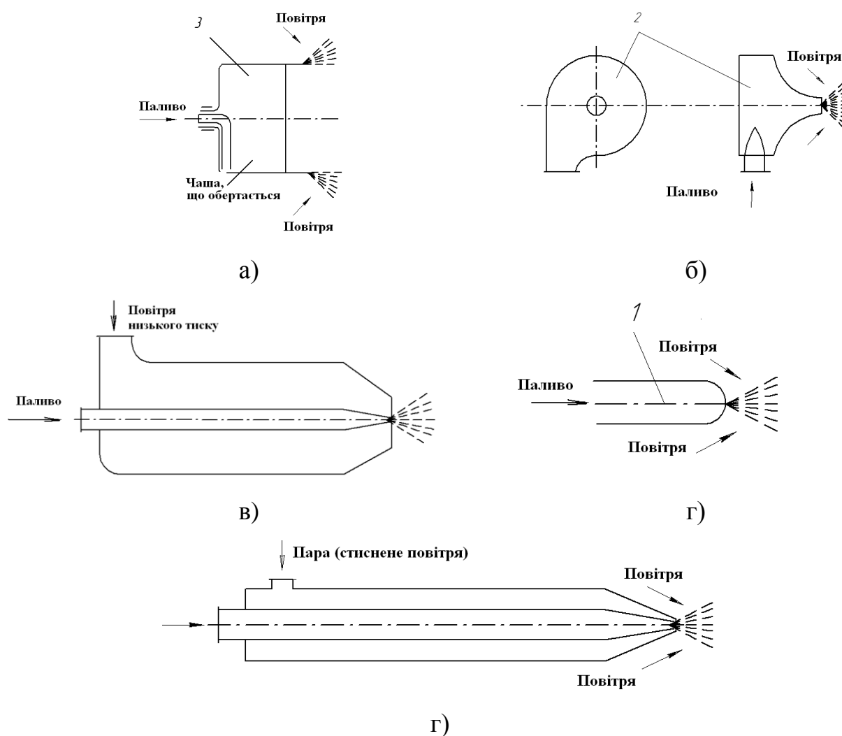
Рис. 3.6. Конструкції механічних форсунок
