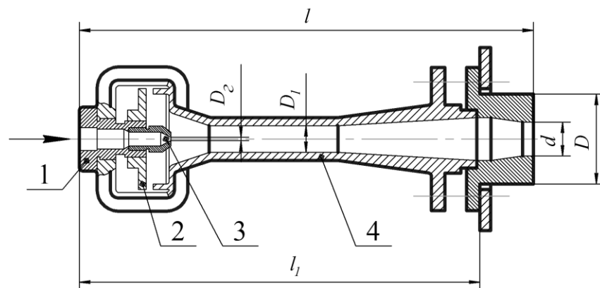
Рисунок 3.11. Інжекційний пальник
