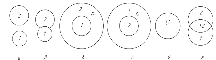
Рис. 1.3. Схема можливих варіантів взаємного розташування зон технологічного процесу (ЗТП) і генерації тепла (ЗГТ).
