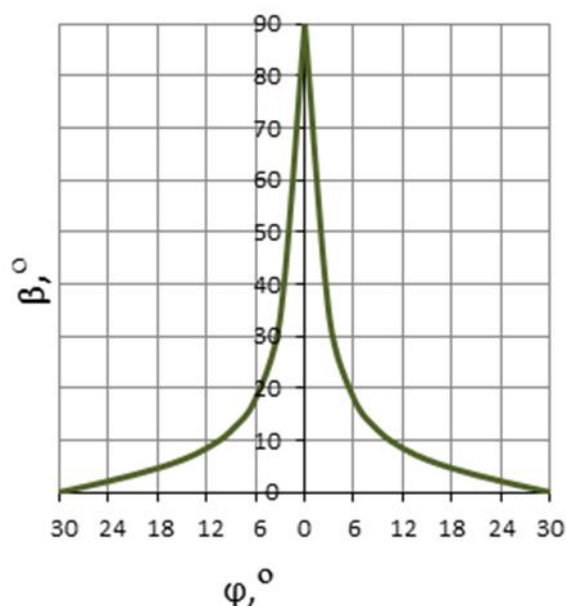
Рис.2 – Кут нахилу фібр \beta в перерізі круглого виробу відносно напрямку плинину суміші у віброекструдері
