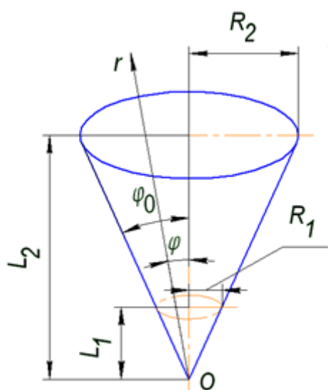
Рис.1 – Розрахункова схема процесу в конічному каналі бункера віброекструдера
