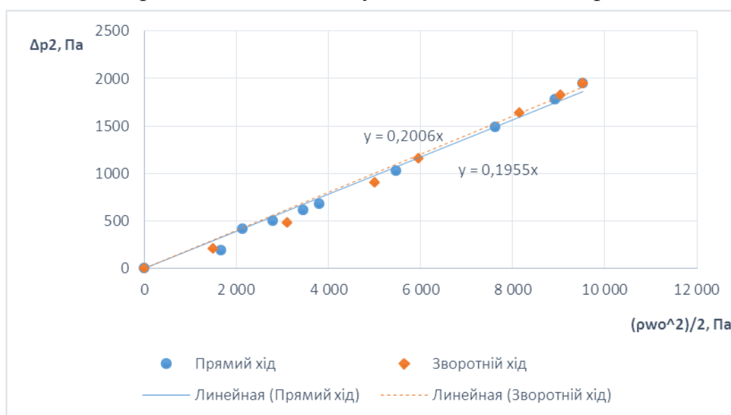
Рисунок 3 – Експериментальна залежність гідралічного опору решітки від гідродинамічного тиску за швидкістю в живому перерізі
