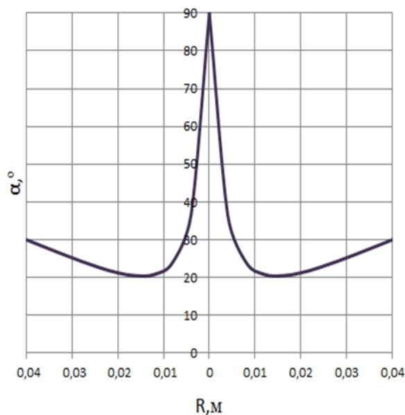
Рис.3 – Кут нахилу фібр \alpha по товщині круглого виробу з радіусом R відносно напрямку формування
