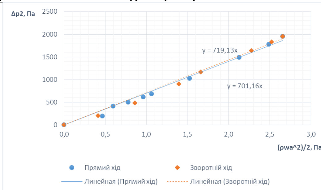
Рисунок 2 – Експериментальна залежність гідралічного опору решітки від гідродинамічного тиску за швидкістю в апараті
