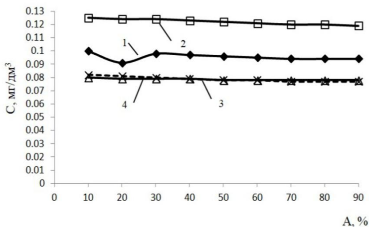
Рис. 1 - Залежність концентрації іонів міді (1), кадмію (2), свинцю (3, 4) від ступеня відбору перміату (А) при фільтруванні розчинів через мембрану ОПМН-П при робочому тиску 0,3 МПА при рН 2,66 (3); 6,20 (1; 2; 4) ( C_{K1} = 0,154 мг/дм 3 ; C_{K2} = 0,131 мг/дм 3 ; C_{K5} = 0,084 мг/дм 3 ; C_{K4} = 0,091 мг/дм 3 )
