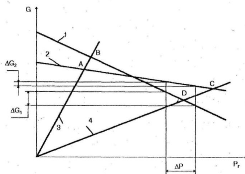
Рисунок 1 – Робочі характеристики екструдера
